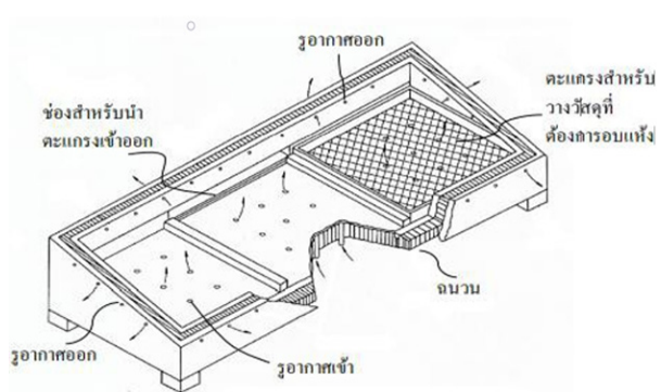
ภาพ 1 ลักษณะของตะแกรงอบแห้ง แบบตู้
