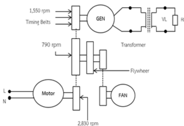
ภาพ 2 หลักการทำงานของพัฒนาระบบอากาศยานผลิตพลังงานไฟฟ้า
